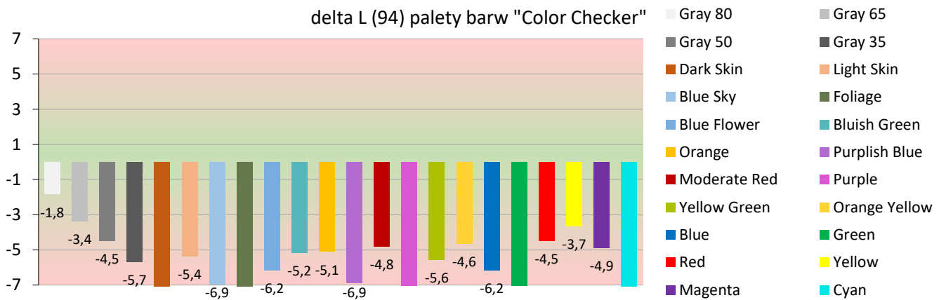
Walidacja względem EBU 3213-E (CIE1960)
